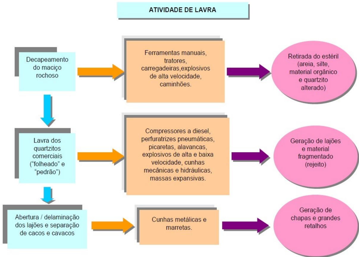
Figura 09 – Fluxograma das Atividades de Lavra do Quartzito
