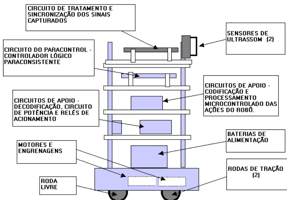
Figura 4.1 – Destaque das partes principais do robô Emmy
