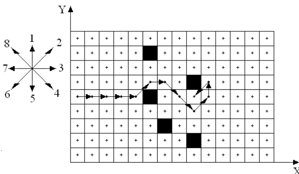
Figura 6.41 Exemplo 8: existem obstáculos nas células (5, 4), (5, 7), (6, 2), (8,1) e (8, 5)
