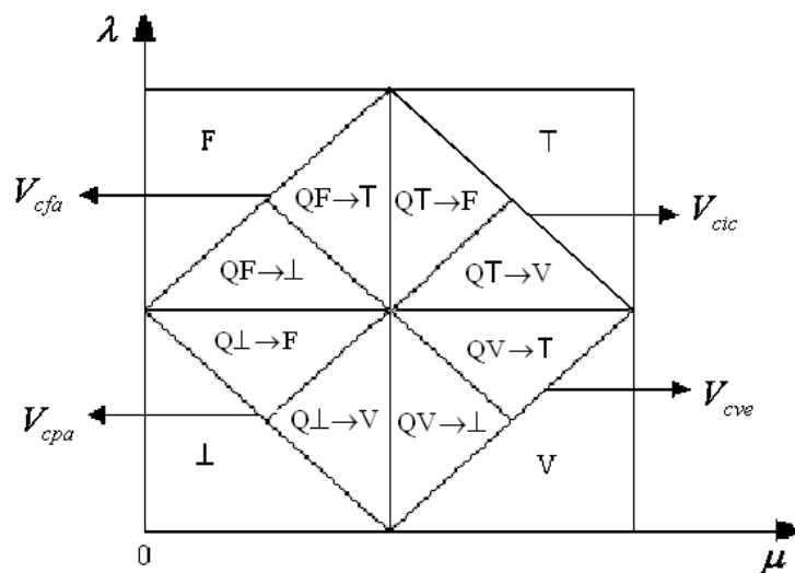
Figura 2.2 Algoritmo paranalizador
