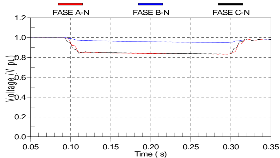
Figura 5. 25 – Evolução temporal da tensão RMS de P7 - Simulação.
