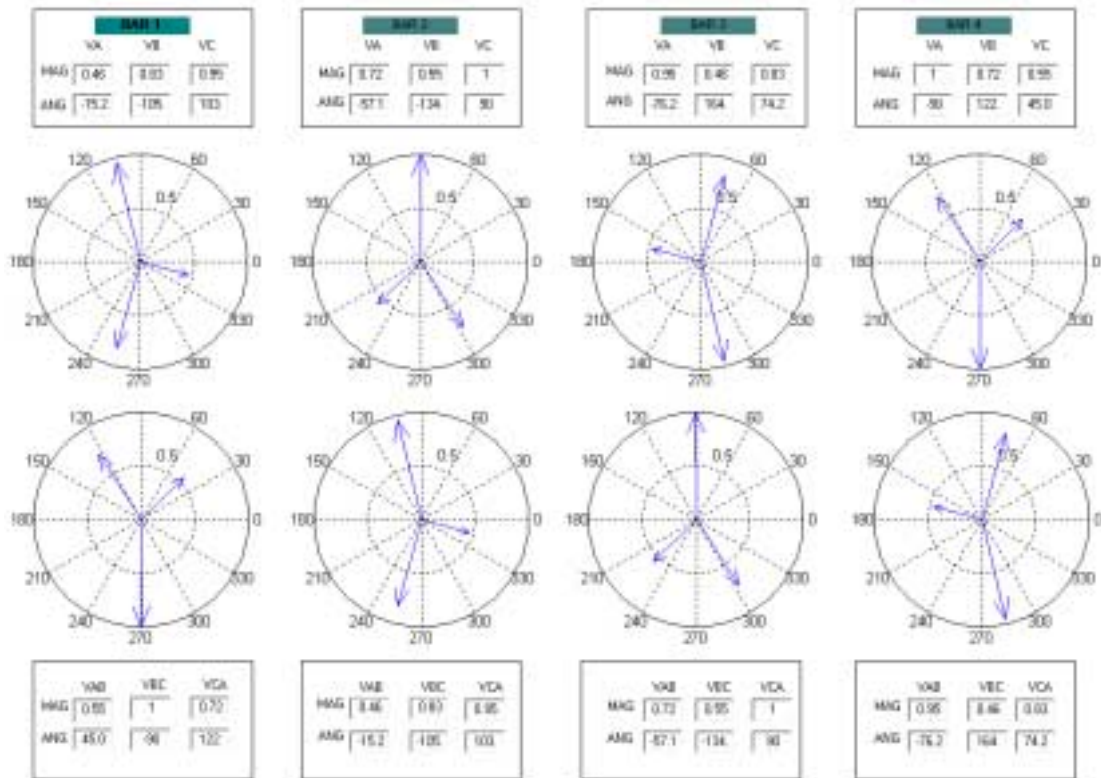
Figura 2. 16 – Sistema Teste – Fasores de tensão nas barras.
