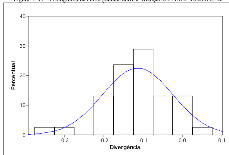
Figura 4.47 – Histograma das divergências entre a Medição e o ANAFAS com 40 \Omega .
