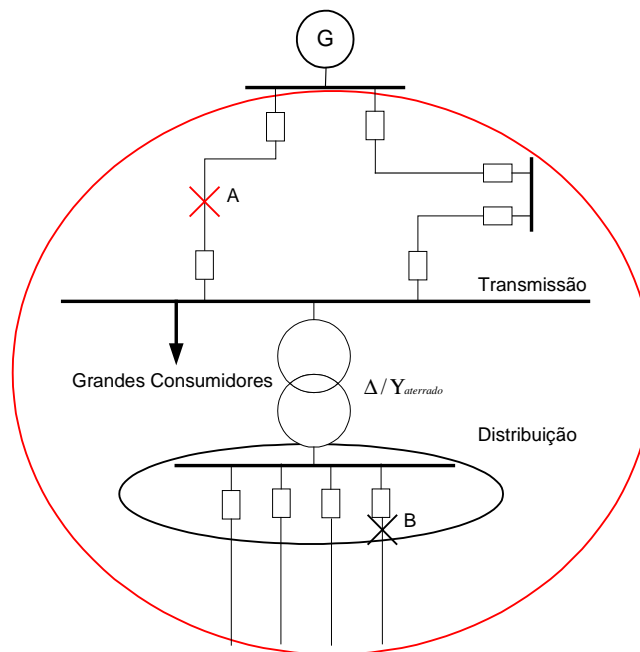
Figura 2. 7 – Área de influência da localização da falta.
