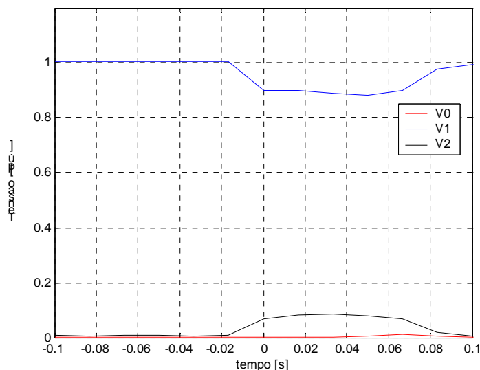
Figura 5. 34 – Evolução temporal das componentes de seqüência da tensão em P8 - Medição.
