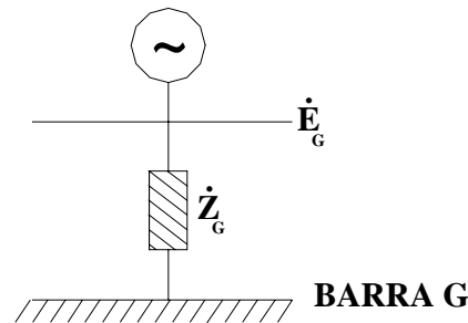
Figura 3. 4 - Representação de gerador - seqüência positiva
