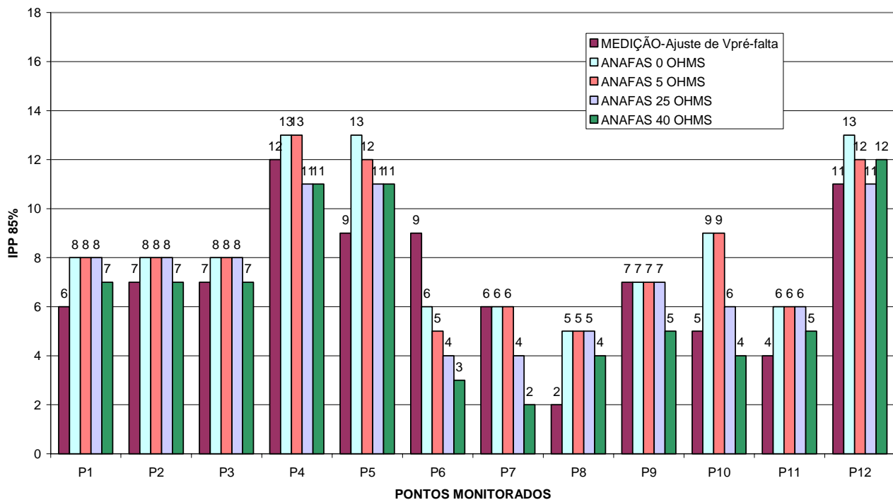
Figura 5. 5 – IPP 85% com variação da resistência de falta-ANAFAS.
