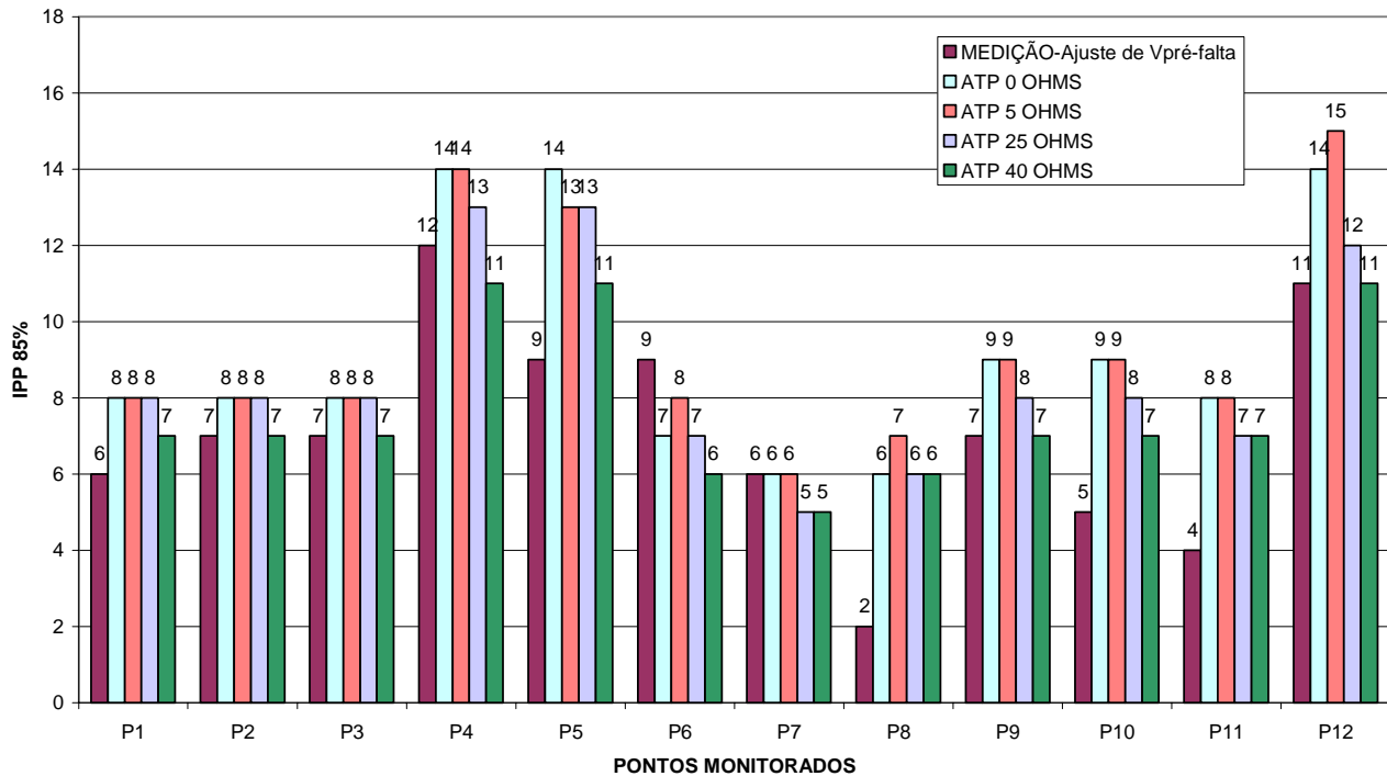
Figura 5. 4 – IPP 85% com variação da resistência de falta - ATP.
