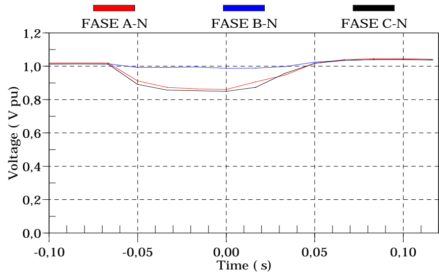
Figura 5. 20 – Evolução temporal da tensão RMS de P6 - Medição.
