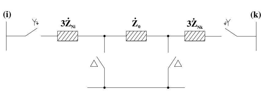
Figura 3. 8 – Representação de transformador de dois enrolamentos - seqüência zero
