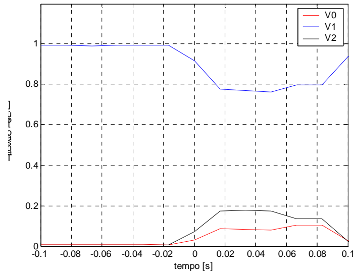
Figura 5. 52 – Evolução temporal das componentes de seqüência da tensão em P4 - Medição.
