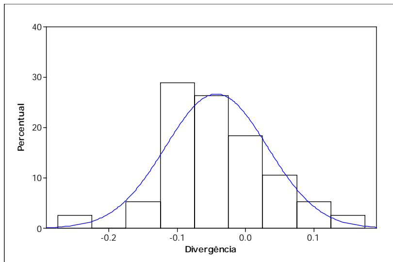
Figura 4.44 – Histograma das divergências entre a Medição e o ATP com 25 \Omega .
