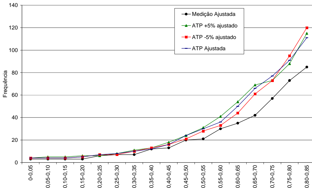
Figura 5. 14 – Frequências acumuladas da intensidades via ATP.
