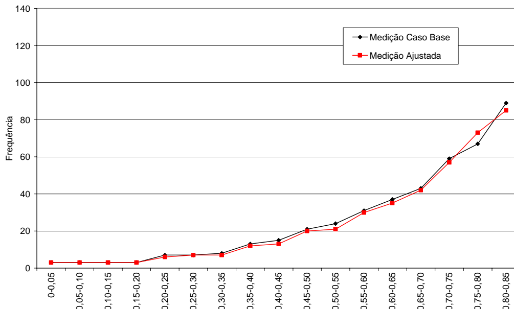
Figura 5. 11 – Freqüência acumulada das intensidades dos afundamentos de tensão via medição.
