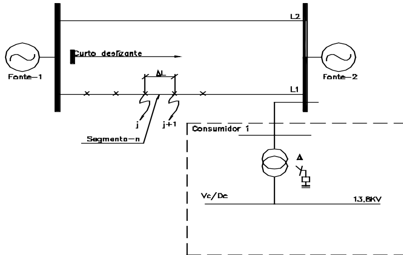
Figura 3. 3 - Diagrama unifilar, método do curto-deslizante.
