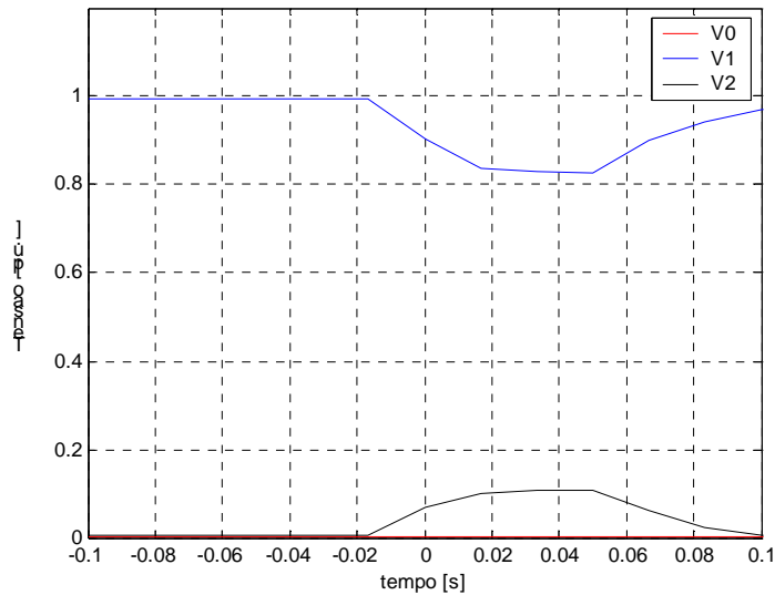
Figura 5. 37 – Evolução temporal das componentes de seqüência da tensão em P11 - Medição.
