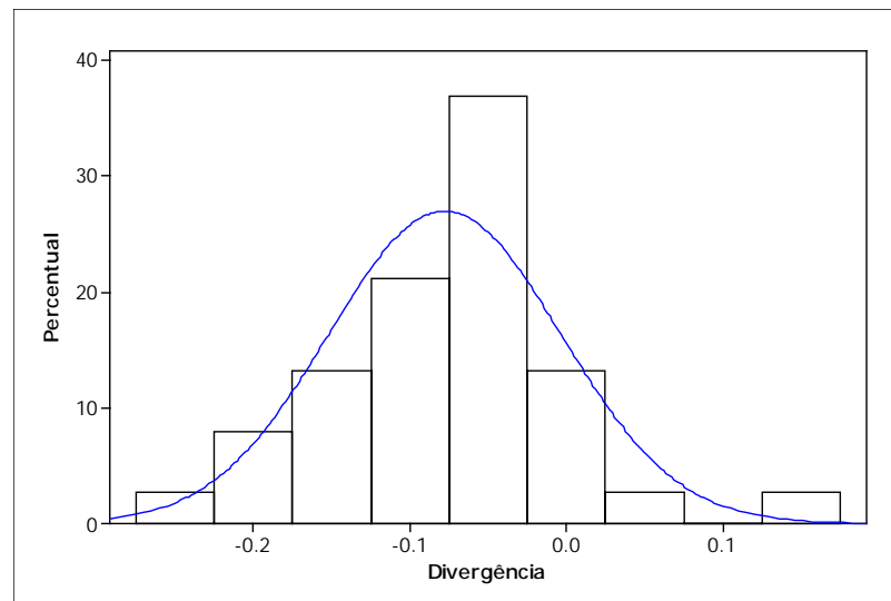
Figura 4.45 – Histograma das divergências entre a Medição e o ANAFAS com 25 \Omega .
