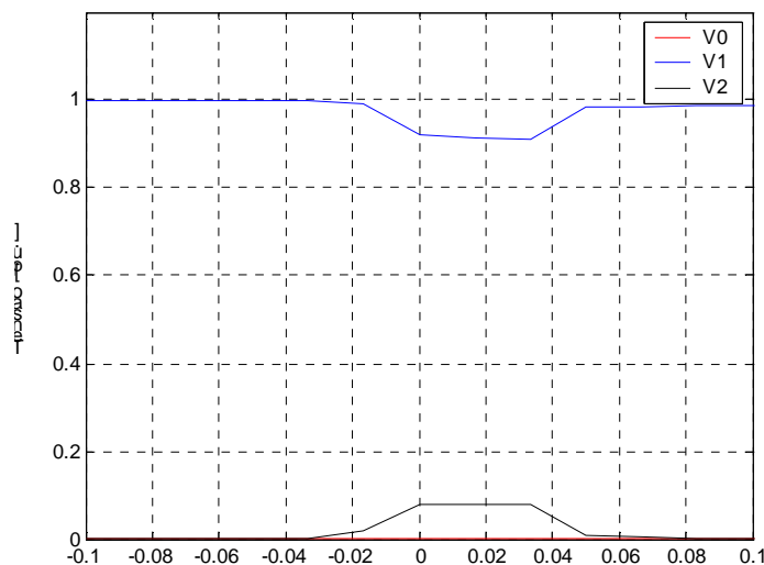
Figura 5. 54 – Evolução temporal das componentes de seqüência da tensão em P12 - Medição.
