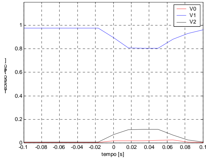
Figura 5. 36 – Evolução temporal das componentes de seqüência da tensão em P10 - Medição.
