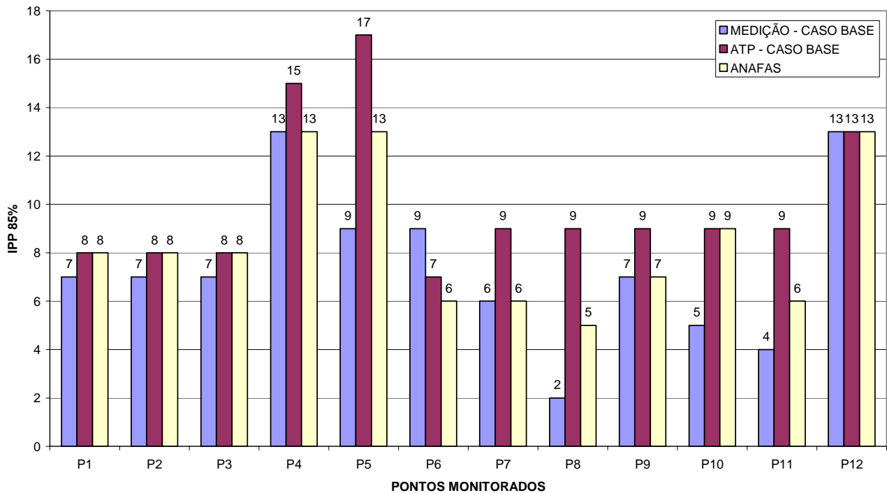
Figura 5. 1 – IPP 85% - Caso Base.
