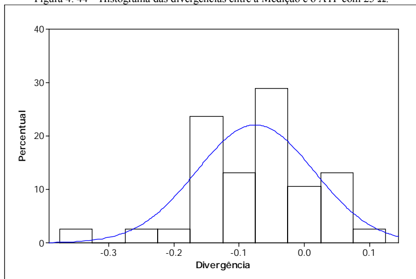
Figura 4.46 – Histograma das divergências entre a Medição e o ATP com 40 \Omega .
