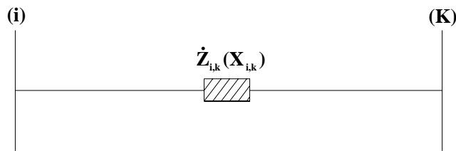
Figura 3. 7 – Representação de transformador de dois enrolamentos - seqüência positiva.
