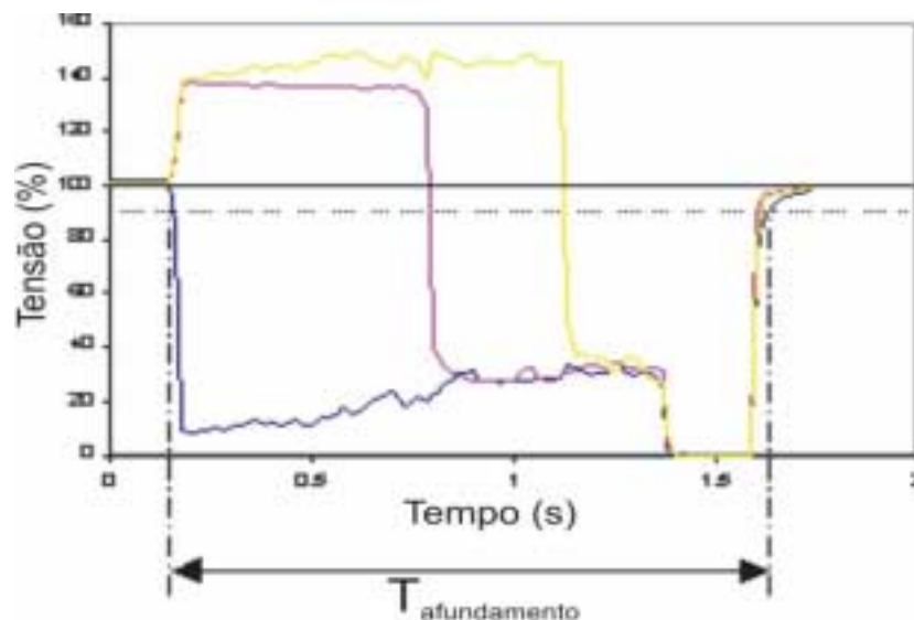
Figura 2. 4 - Caracterização de afundamentos de tensão segundo a UNIPEDA.
