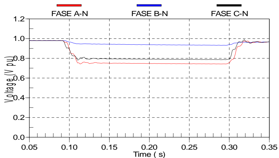
Figura 5. 23 – Evolução temporal da tensão RMS de P9 - Simulação.
