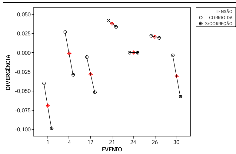
Figura 4. 16 – Influência da tensão pré-falta nas divergências entre medição e ATP em P1.
