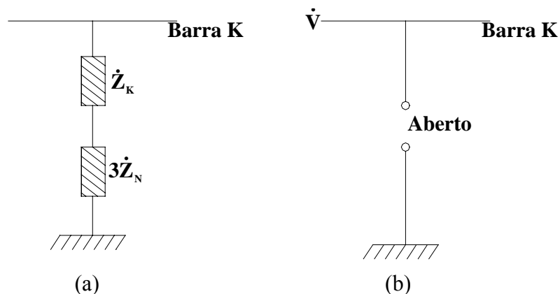
Figura 3. 14 - Representação de capacitor e reator de barra - seqüência zero
