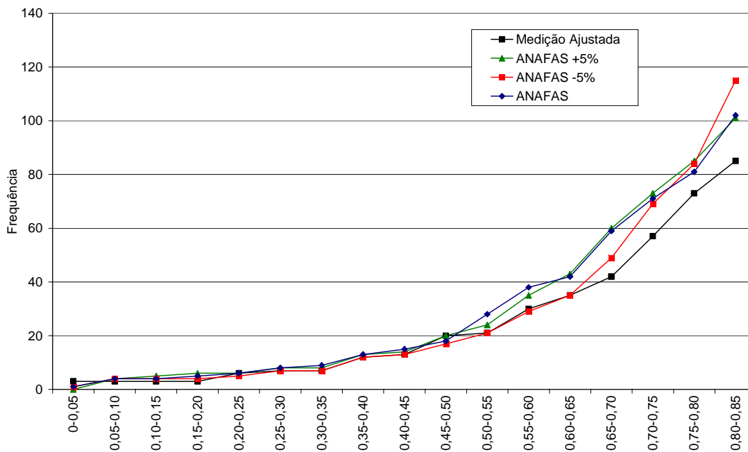
Figura 5. 15 – Frequências acumuladas da intensidades via ANAFAS.
