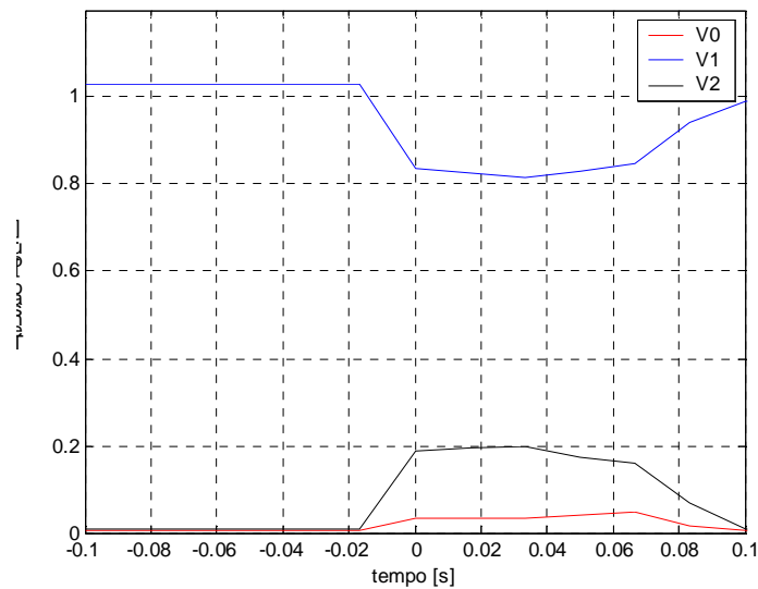
Figura 5. 53 – Evolução temporal das componentes de seqüência da tensão em P5 - Medição.
