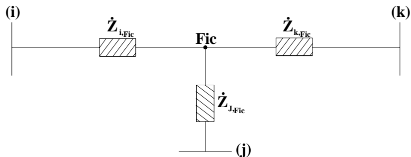
Figura 3. 9 – Representação de transformador de três enrolamentos - seqüência positiva.
