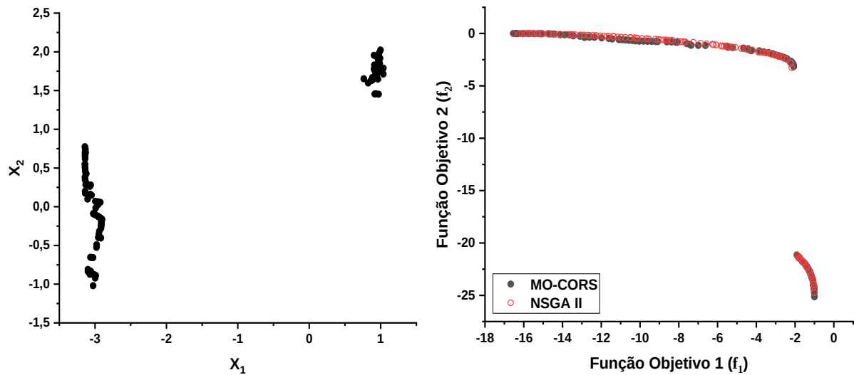
Figura 4.9: Espaço de decisão e frente de Pareto MOP3.
