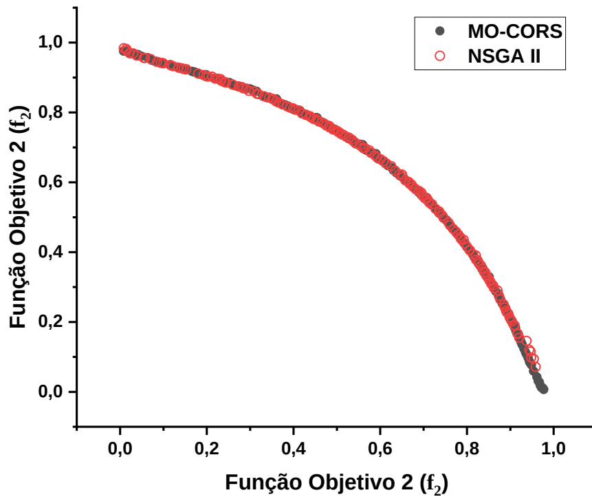
Figura 4.21: Frentes de Pareto do problema ZDT2 (6 variáveis).
