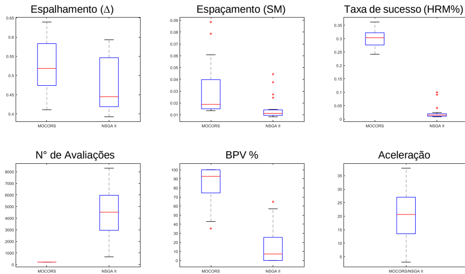
Figura 4.20: Métricas e aceleração para o problema ZDT2 (6 variáveis).
