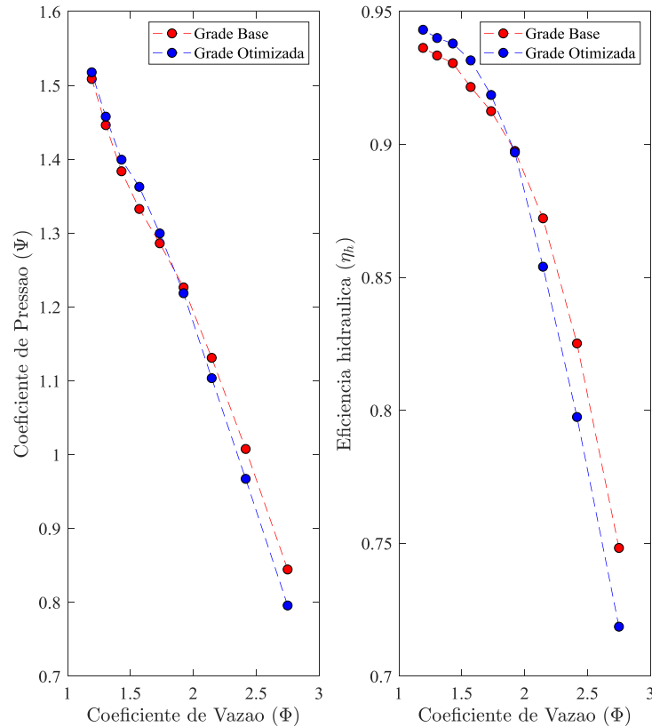
Figuras 5.27: Curvas de desempenho operacional das grades.
