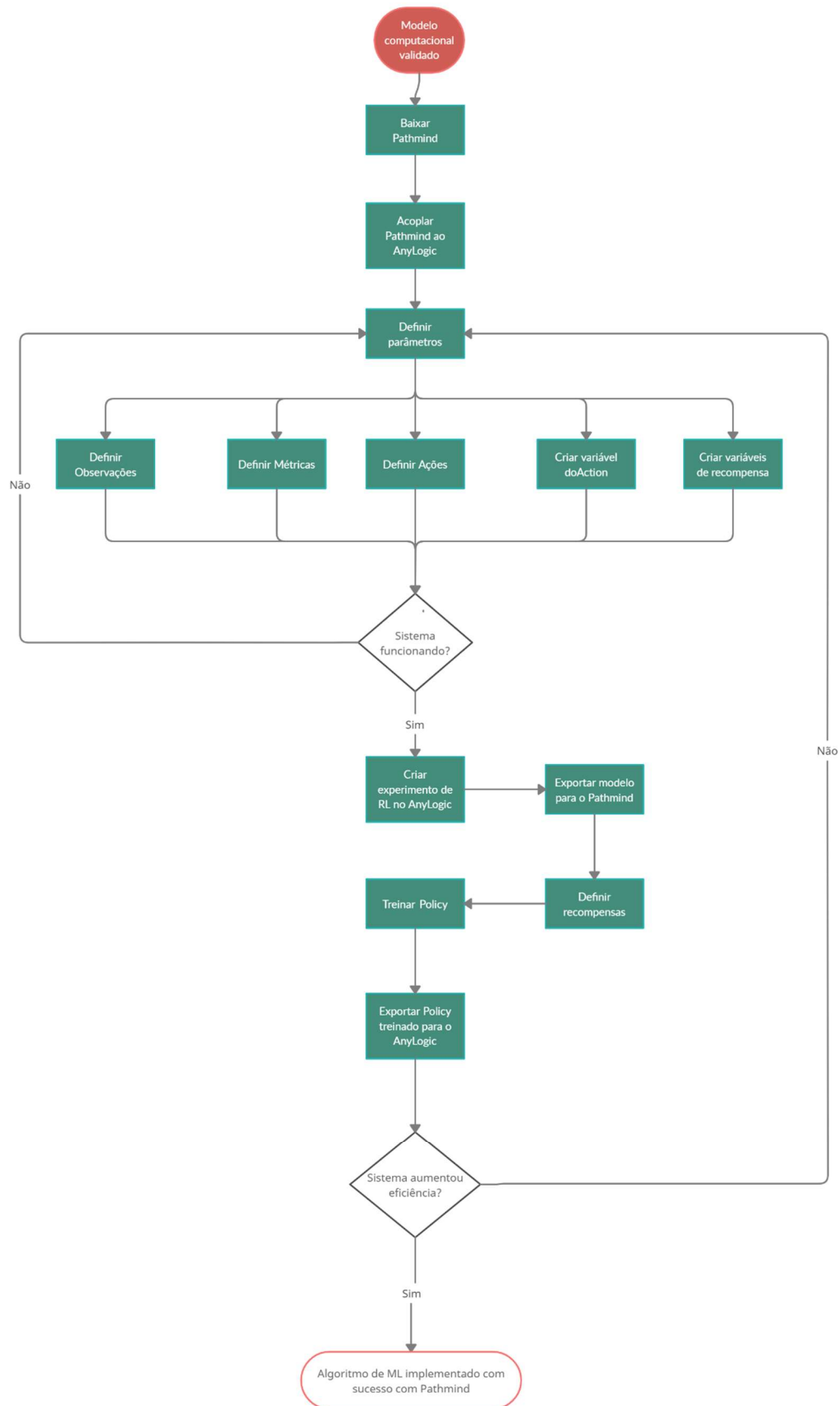
Figura 19 - Fluxograma de implementação do ML utilizando Pathmind Fonte: Autor
