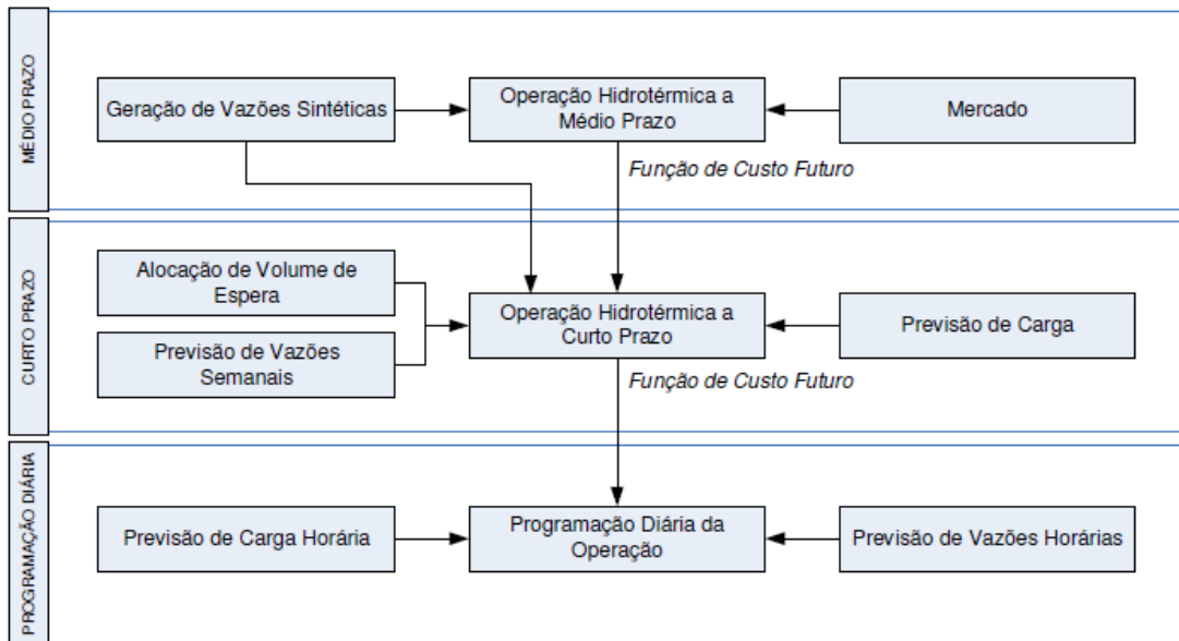
Figura 6 - Planejamento da operação energética atual
